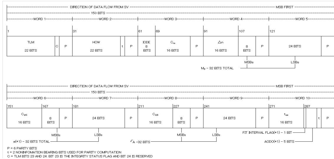
Figure 4.1.2-3 Subframe 2 Format
